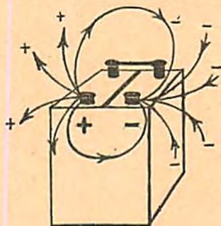
Fig. 9. — Aspect de la pile électrique et du réseau de forces électriques qui relie le pôle positif au pôle négatif à travers l'universion. Lorsque aucun conducteur ne relie extérieurement les pôles, la pile est à l'état d'équilibre statique.
