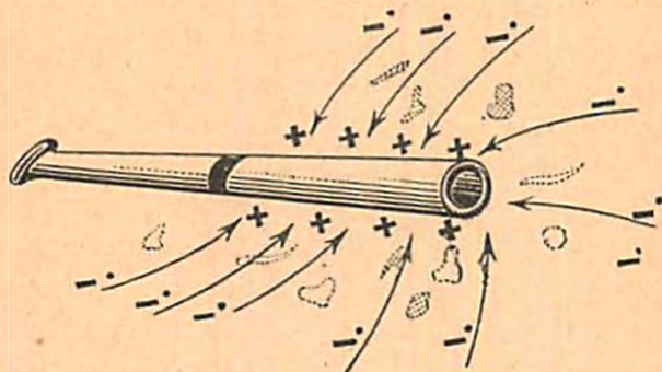
Fig. 5. — En frottant le fume-cigarette d'ambre, on lui enlève une certaine quantité d'universon, c'est-à-dire d'électrons ou de grains d'électricité négative. Autrement dit, on charge positivement le fume-cigarette. Les électrons négatifs accourent du dehors pour neutraliser cette électrisation et entraînent dans leur course les objets légers, papiers et fétus, qui se précipitent sur le fume-cigarette.
